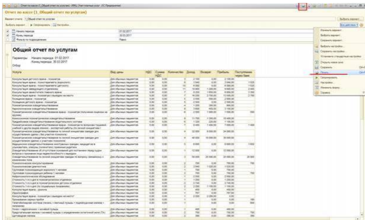
Рисунок 136 Печать отчета
