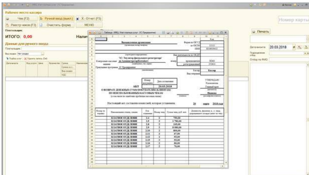
Рисунок 131 Акт возврата
