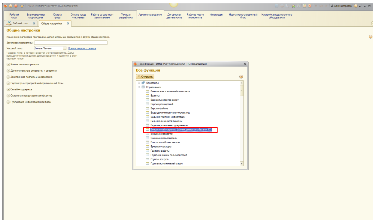
Рисунок 1 Настройка подключения
