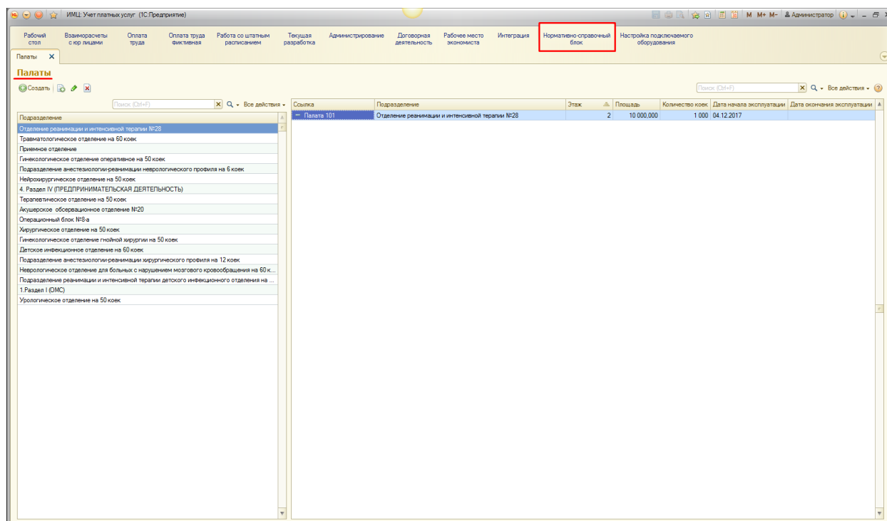
Рисунок 7 Справочник «Палаты»
