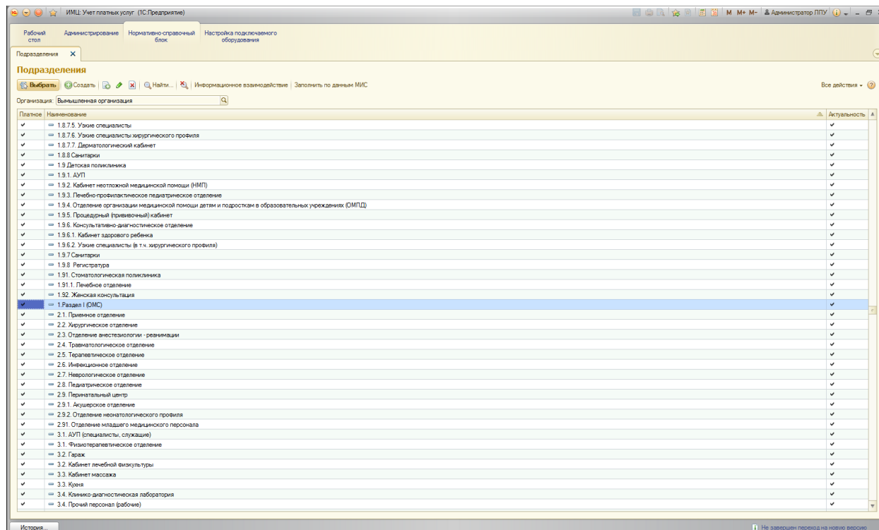
Рисунок 1 Справочник «Подразделения»
