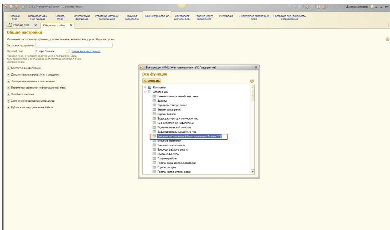
Рисунок 1 Настройка подключения
